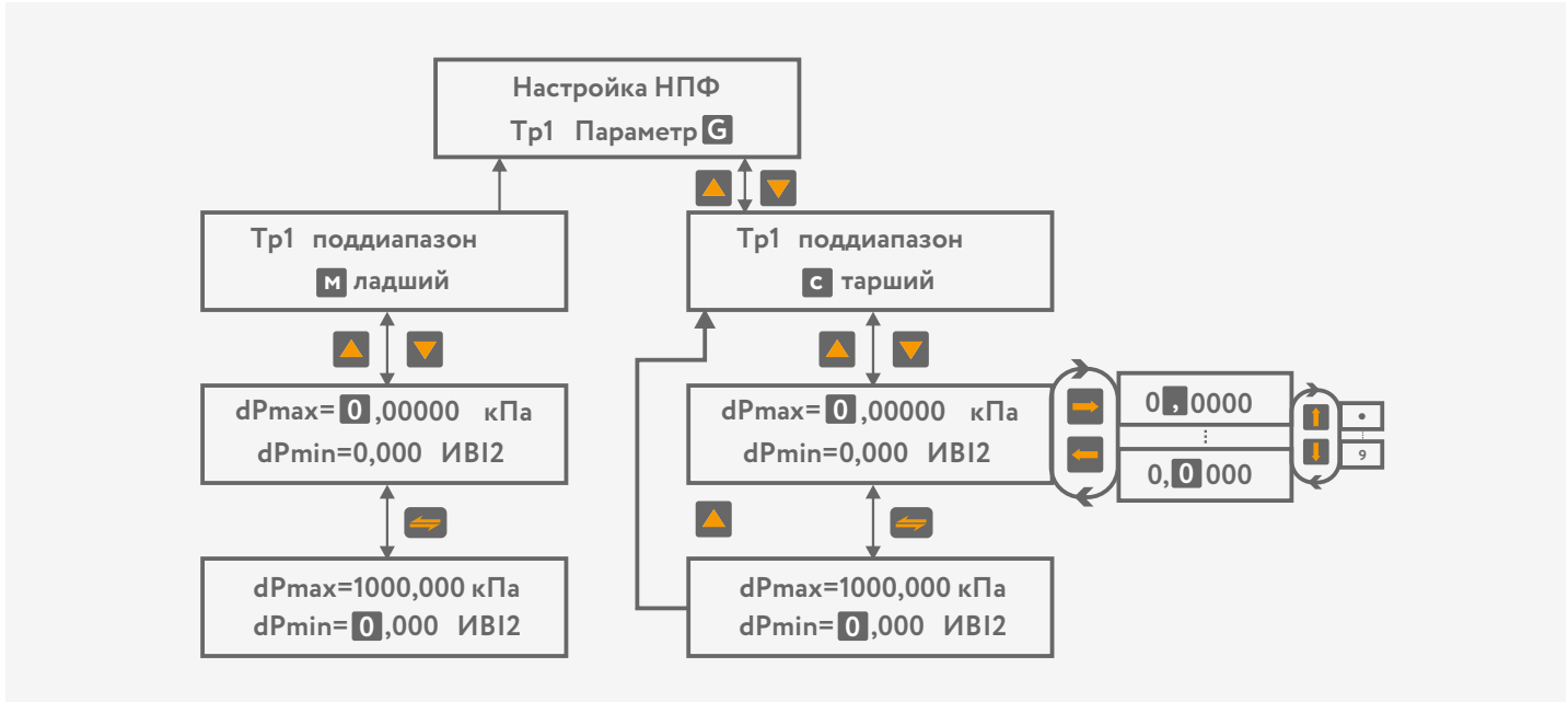
Рисунок 6.5. Настройка НПФ для расходомера переменного перепада
