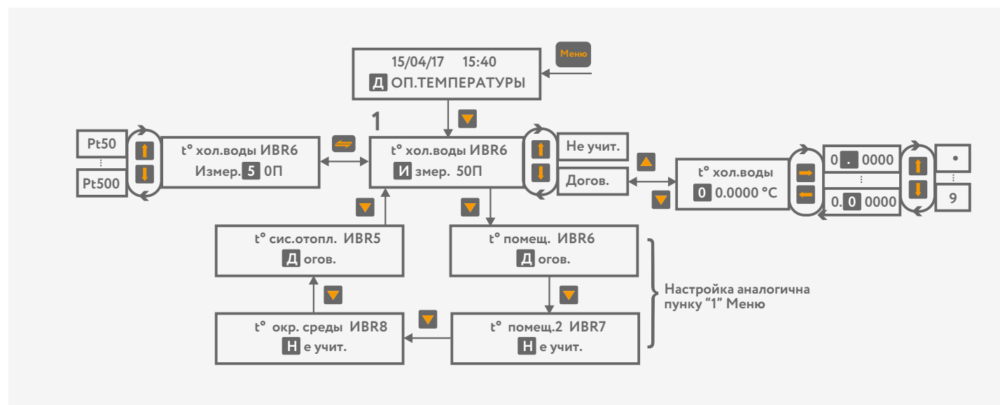
Рисунок 9 – Выбор условий измерений и порядок настройки каналов доп. температур.
