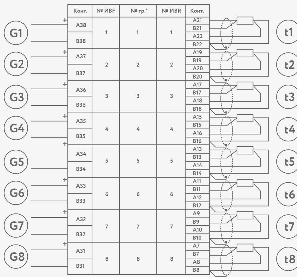
Виды выходных цепей датчиков расхода G1...G8
