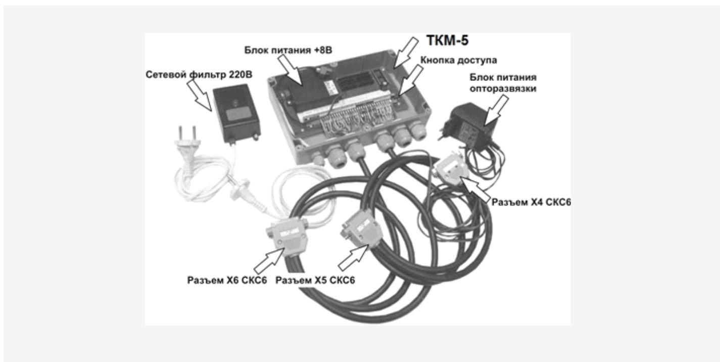
Рис. Б.3 Внешний вид ТКМ-5 Технологический коммутационный модуль ТКМ-5 поставляются изготовителем вычислителя по отдельному заказу.
