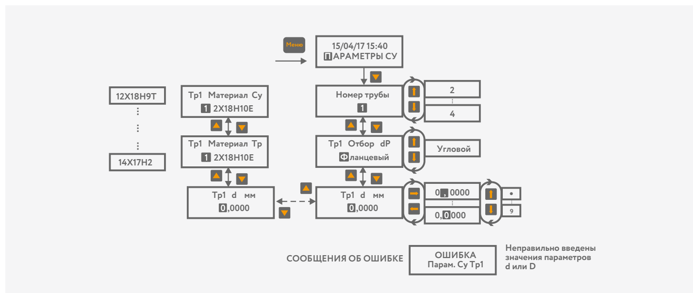
Рисунок 5 – Последовательность действий по установке параметров СУ
