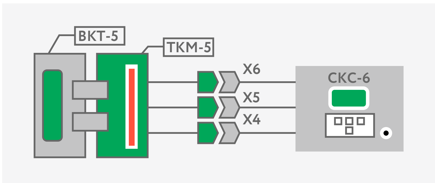
Рис. Б.2 Схема поверки ВКТ-5 с использованием СКС-6 и ТКМ-5 Разъемы X4...X6 (ТКМ-5) подключаются к одноименным разъемам стенда СКС6
