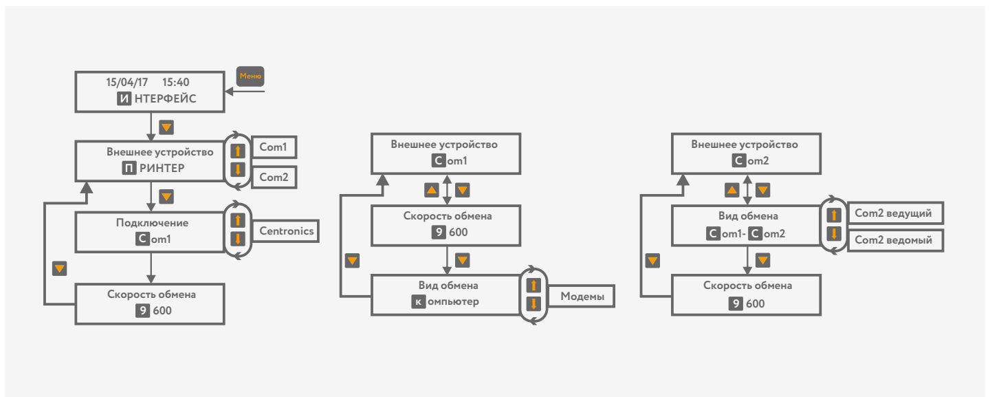
Рисунок 10 – Установка параметров интерфейса
