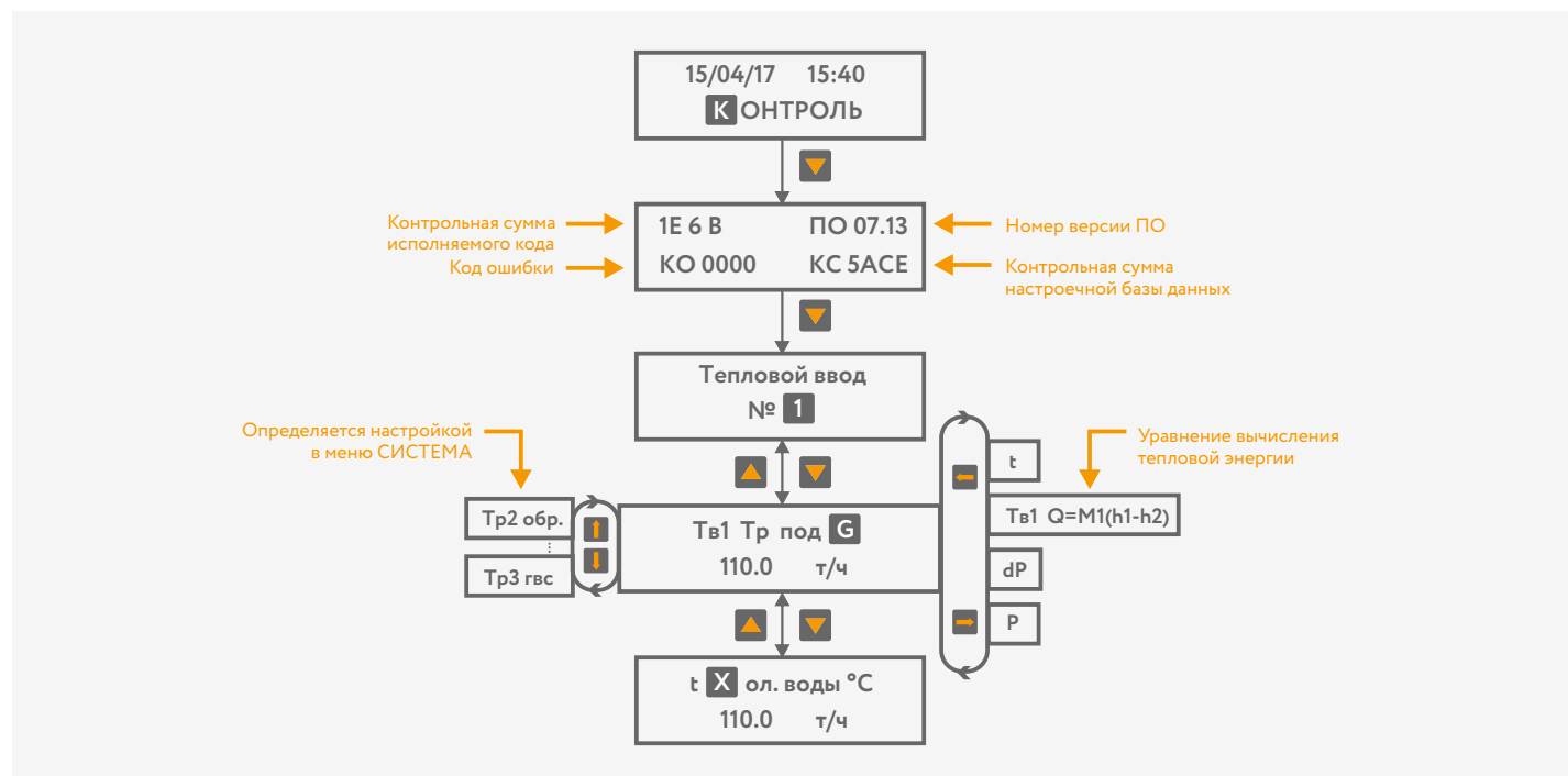
Рисунок 17 – Порядок действий по просмотру текущих параметров теплоносителя
