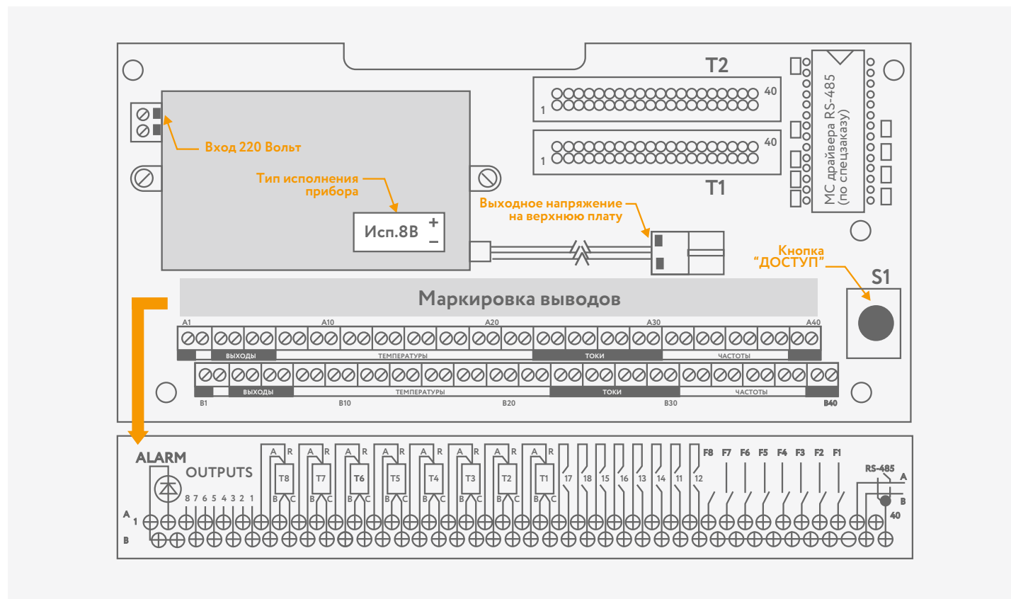
Рисунок 2 – Внешний вид платы клеммников
