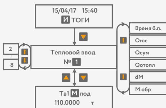
Рисунок 18 – Порядок действий по просмотру информации на дисплее
