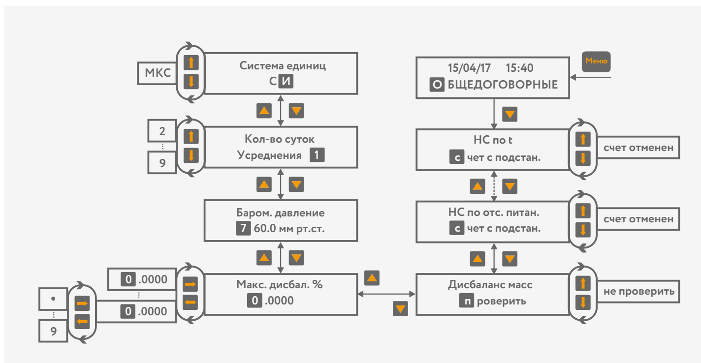
Рисунок 8 – Установка общедоговорных параметров
