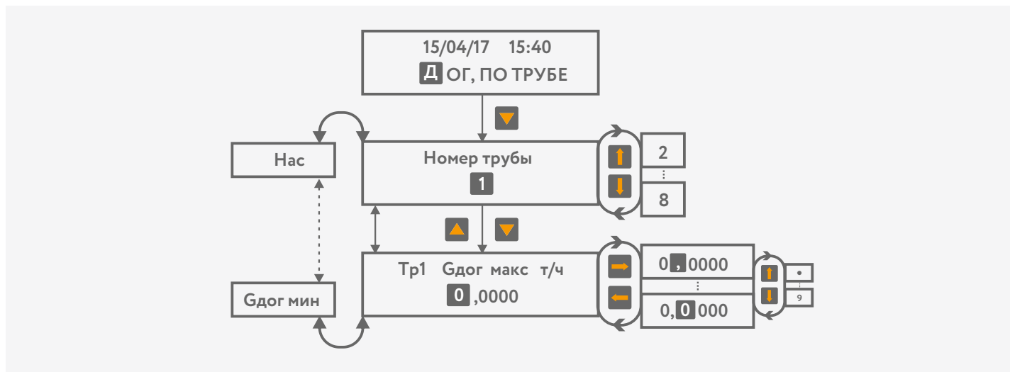
Рисунок 7 – Установка договорных параметров по трубопроводам
