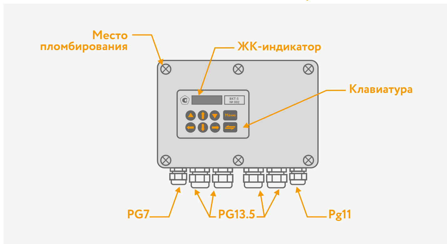
Рисунок 1 – Внешний вид вычислителя
